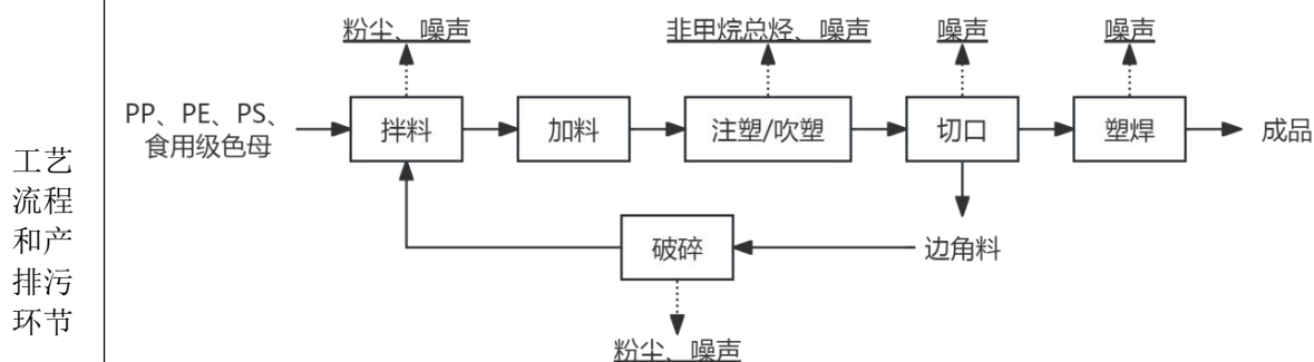
图 2-2 项目工艺流程图
