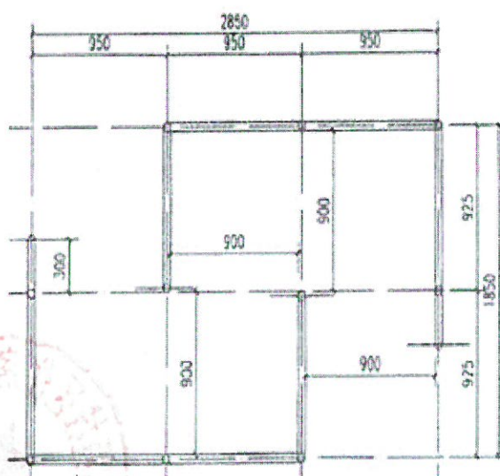
图 1 双 C 通道平面图
