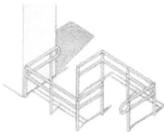
图 3 双 C 通道立面图 2
